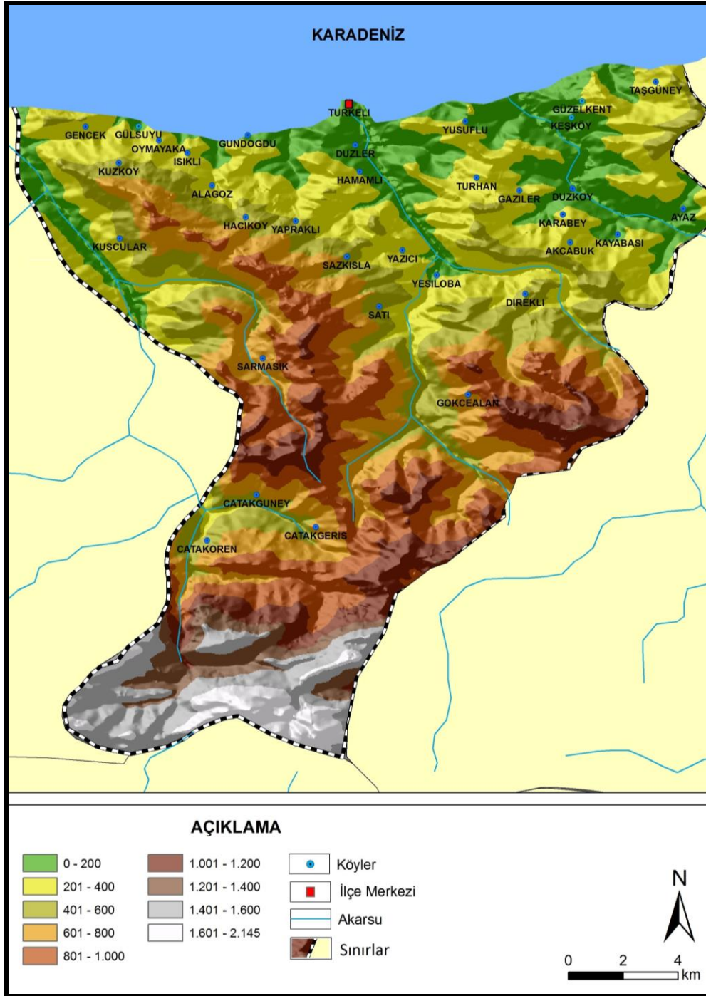
Şekil 2. Türkeli ilçesi topografya haritası.
