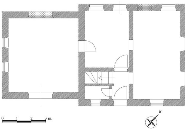
Çizim 32: Hamzalı İstasyonu Zemin Kat Planı
