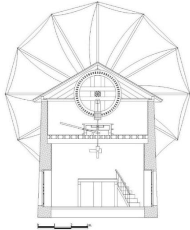
Çizim 23: Çırakman Yel Değirmeni Kesiti (Belediye Arşivi'nden İşlenerek)
