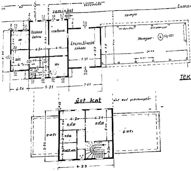
Çizim 27: Tekkeköy İstasyon Binası İlk Planı (Tekkeköy Belediye Arşivi)
