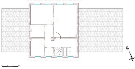
 izim 29: Tekkek y İstasyon Binası Birinci Kat Planı (Tekkek y Belediyesi Arşivi'nden İ lenerek)
