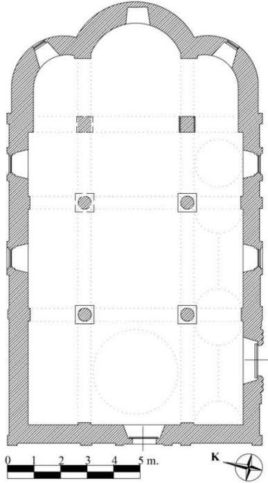
Çizim 44: Asarağaç (Kelkaya) Kilisesi Planı
