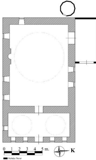
Çizim 50: Karaperçin Kilise Camii Planı
