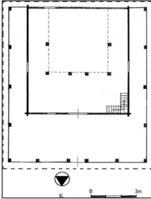
 izim 3: Tekkek y  Sarıyurt K y  Ah ap Camii Planı (E y p Nefes, Tekkek y  Y resi'nde  antı Tekni inde İ a Edilen Ah ap Camiler, s. 125)
