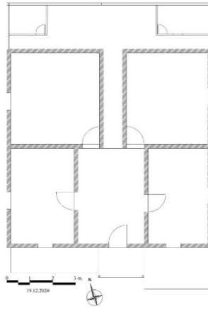
 izim 37:  ayır kek K y  2 Nolu Evin Planı
