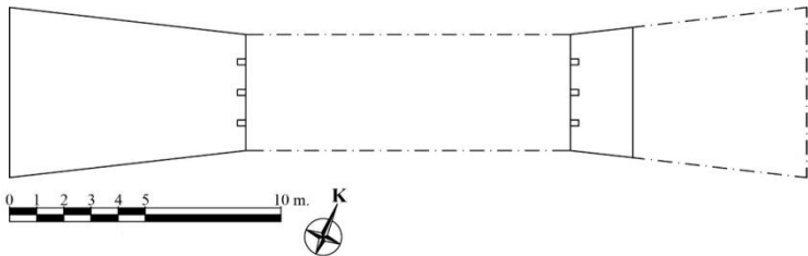
Çizim 16: Tekkeköy Çayırçökek Köprüsü Planı
