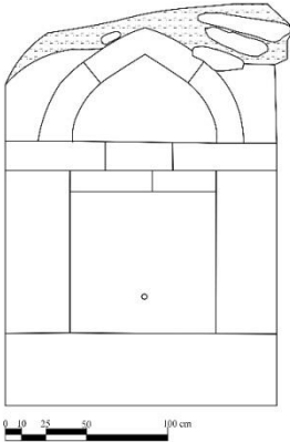
 izim 13: Tekkek y Kazancılı  eşmesi Cephe  izimi
