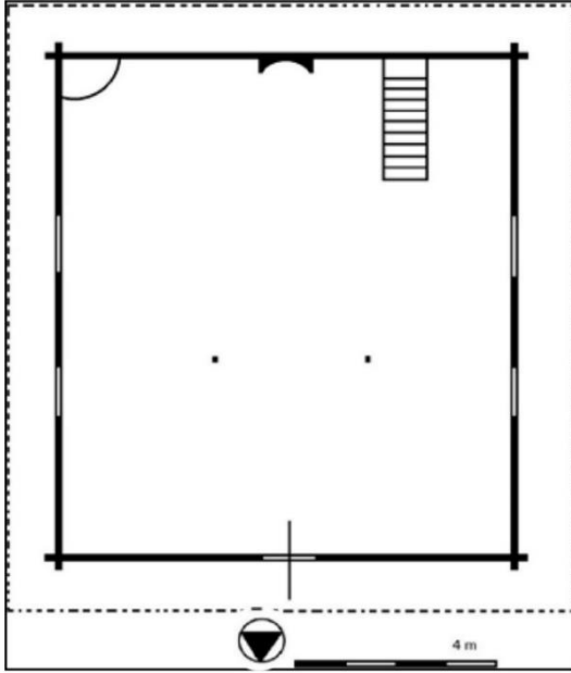
 izim 5: Tekkek y  Yeşildere K y  Ahşap Camii Planı (Ey p Nefes, Tekkek y  Y resi'nde  antı Tekniğinde İ şa Edilen Ahşap Camiler, s. 134)
