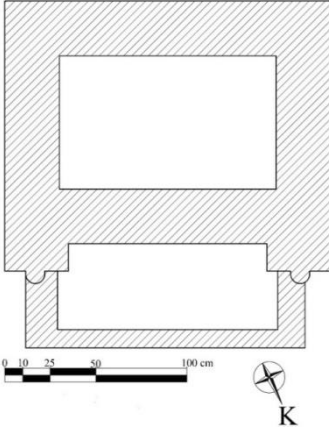
Çizim 9: Tekkeköy Fırıncıoğlu Çeşme Planı
