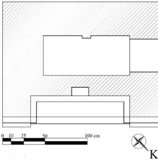
Çizim 7: Tekkeköy Bakacak Çeşmesi Planı
