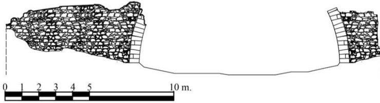
 izim 17: Tekkek y  ayır  kek K pr s  Cephe  izimi
