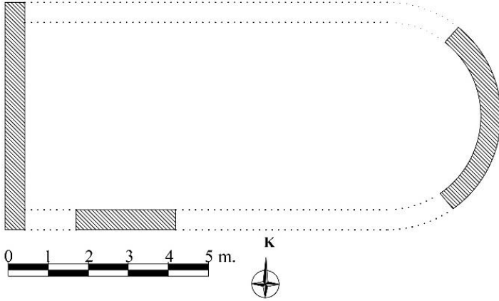
Çizim 51: Yazılar Kilisesi Planı
