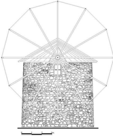
Çizim 22: Çırakman Yel Değirmeni Cephe Görünüşü (Belediye Arşivi'nden İşlenerek)
