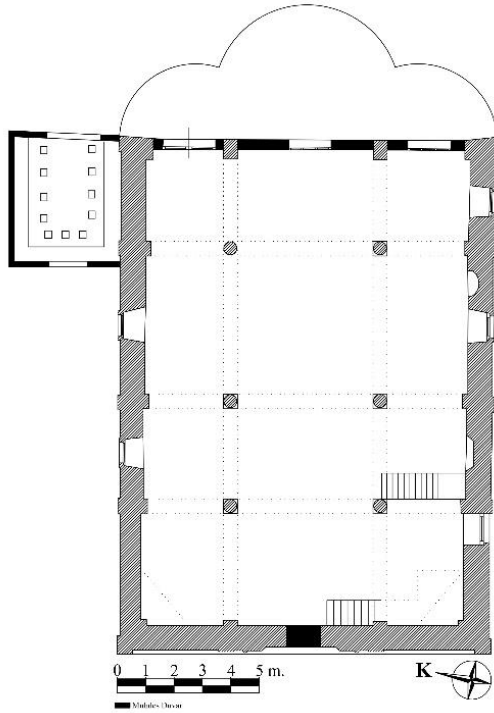
 izim 43: Tekkek y Antyeri (Hagios Demetrios Kilisesi) Camii Planı
