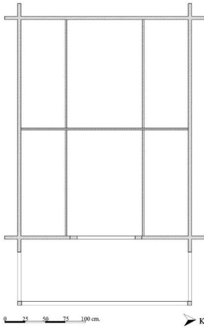
 izim 38: B y kl  Mahallesi  zkan Kaymak'a ait Ambarın Planı
