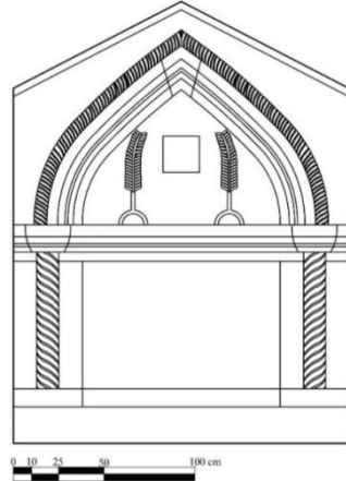
Çizim 10: Tekkeköy Fırıncıoğlu Çeşmesi Restitüsyon Çizimi
