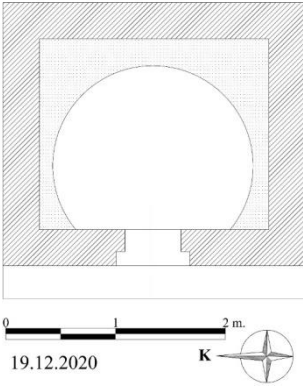
Çizim 41: Sarıyurt 2 No'lu Fırın Planı
