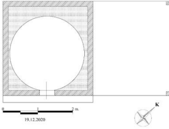
Çizim 39: Sarıyurt-Halburcu 1 No'lu Fırın
