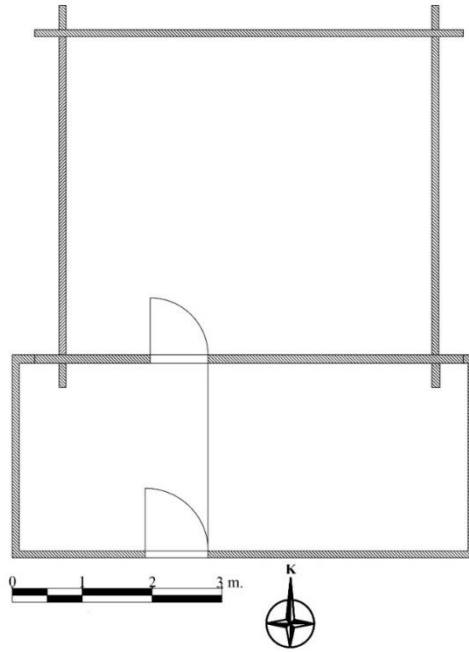
 izim 24: Tekkek y  /  ayır  kek K y  İsmail  ayır  kek Su Değirmeni Planı
