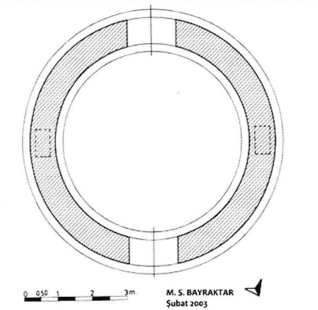
Çizim 19: Tekkeköy Çırakman Yel Değirmeni Planı
