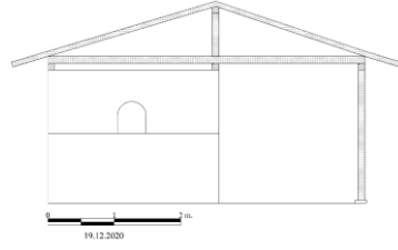
Çizim 40: Sarıyurt-Halburcu 1 No'lu Fırının Cephesi
