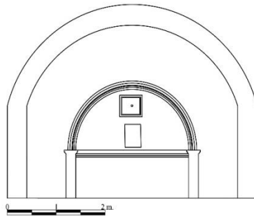
 izim 12: Tekkek y  ırakman Mahallesi    mesi Cephe  izimi
