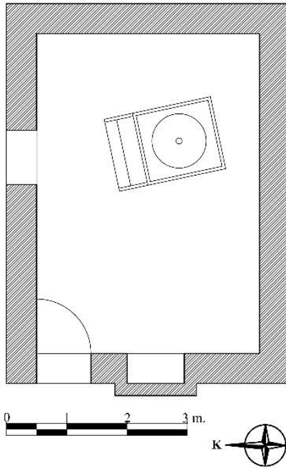
 izim 26: Sarıyurt K y  Halburcu Mahallesi Su Deęirmeni Planı
