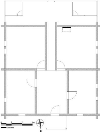
 izim 36:  ayır kek K y  1 Nolu Evin Planı
