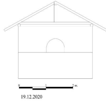
Çizim 40: Sarıyurt-Halburcu 1 No'lu Fırının Cephesi
