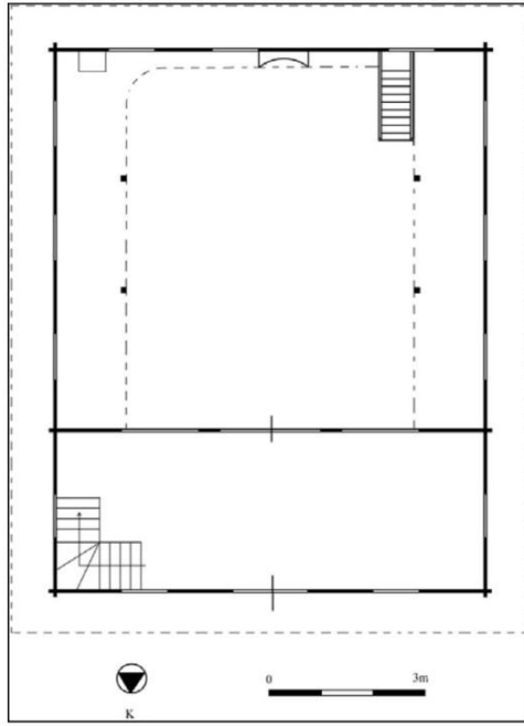
 izim 4: Tekkek y  G zelyurt K y  Ah ap Camii Planı (Ey p Nefes, Tekkek y  Y resi'nde  antı Tekni inde İ a Edilen Ah ap Camiler, s. 117)
