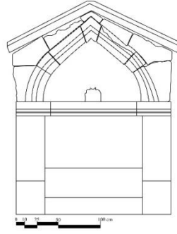
Çizim 8: Tekkeköy Bakacak Çeşmesi Cephe Çizimi
