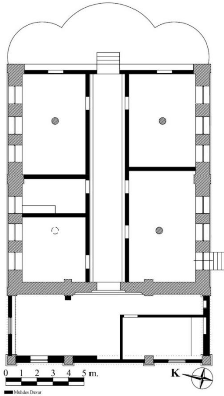
Çizim 45: Aşağıçinik Kilisesi Planı
