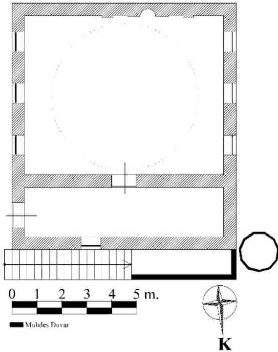
Çizim 49: Çimenli Kilise Camii Planı
