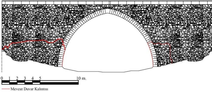
 izim 18: Tekkek y  ayır  kek K pr s  Restit syon  izimi
