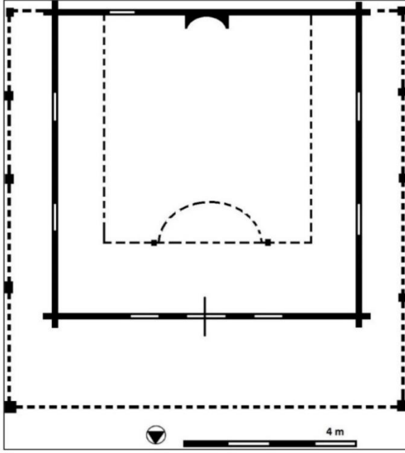
Çizim 2: Tekkeköy Çayırçökek Köyü Ahşap Camii Planı (Eyüp Nefes, Tekkeköy Yöresi'nde Çantı Tekniğinde İnşa Edilen Ahşap Camiler, s. 115)
