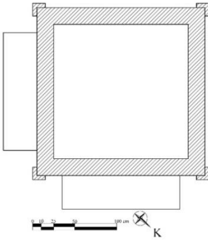
Çizim 15: Tekkeköy Büyüklü Çeşmesi Planı
