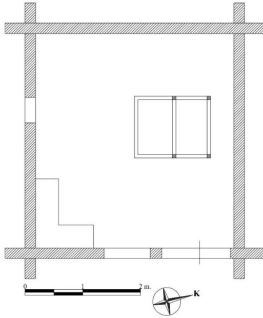
Çizim 25: Tekkeköy Yeşildere Köyü Su Değirmeni Planı
