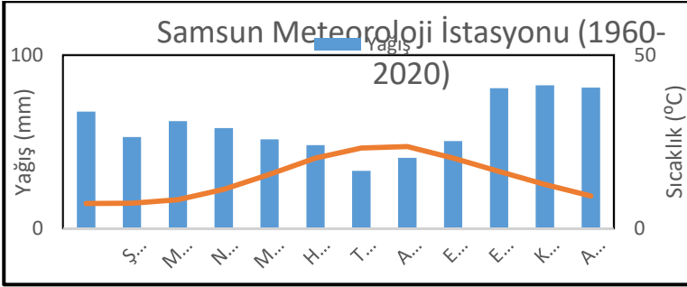
Şekil 4. Samsun Meteoroloji İstasyonu'nun aylık ortalama yağış ve sıcaklık diyagramı.
