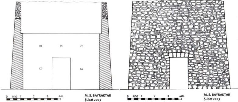
Çizim 20: Çırakman Yel Değirmeni 2003 Öncesi Kesiti
