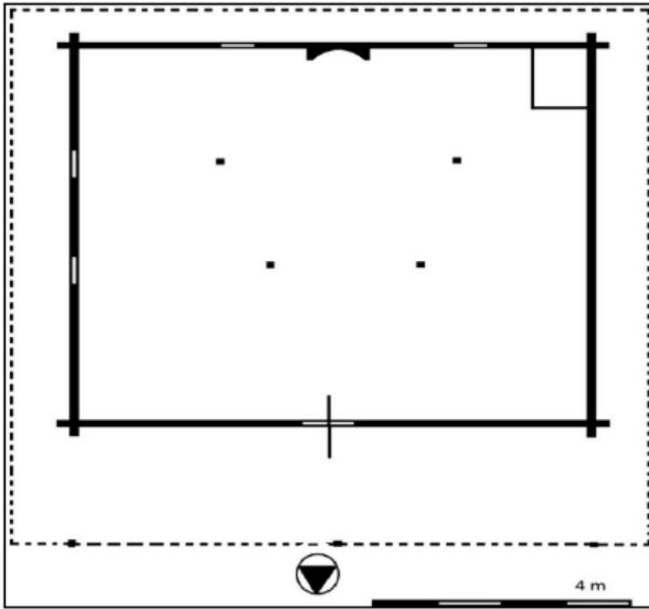
Çizim 6: Tekkek y Yeşilalan K y  Ahşap Camii Planı (Ey p Nefes, Tekkek y Y resi'nde  antı Tekniğinde İnşa Edilen Ahşap Camiler, s. 139)
