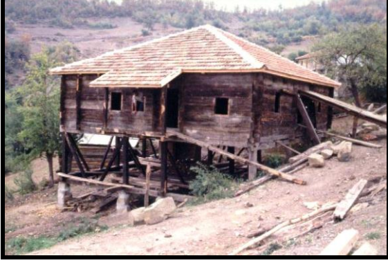
Foto 38,39. Ahşap bir evin sökülerek yeniden inşa edilmesi (Türkeli-Çatak köyü). Sökülmüş bir ahşap evin duvarlarının betonarme bir evin ikinci katında kullanılması, alt kat beton üst kat ahşap, (Çatalzeytin-Paşalı köyü).
